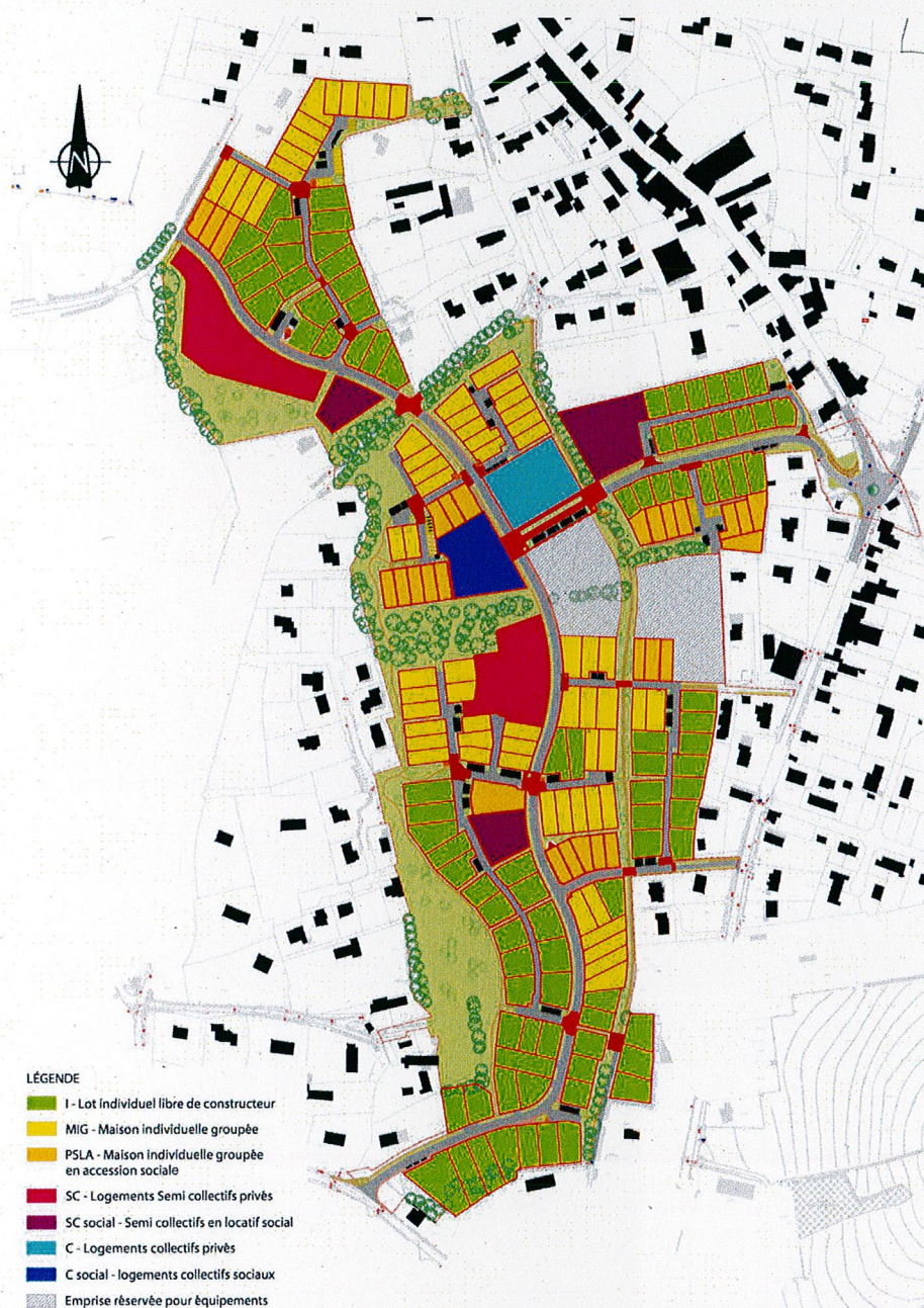
Schéma d'aménagement de la ZAC « les Hauts du Sénéchal » -SETUR décembre 2014
